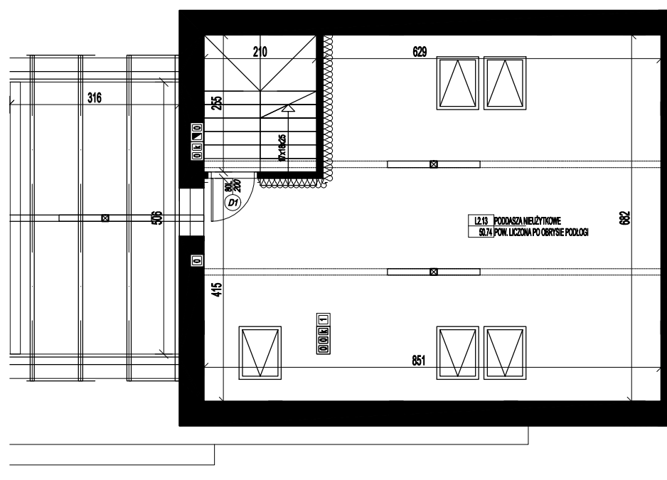
RZUT PODDASZA
