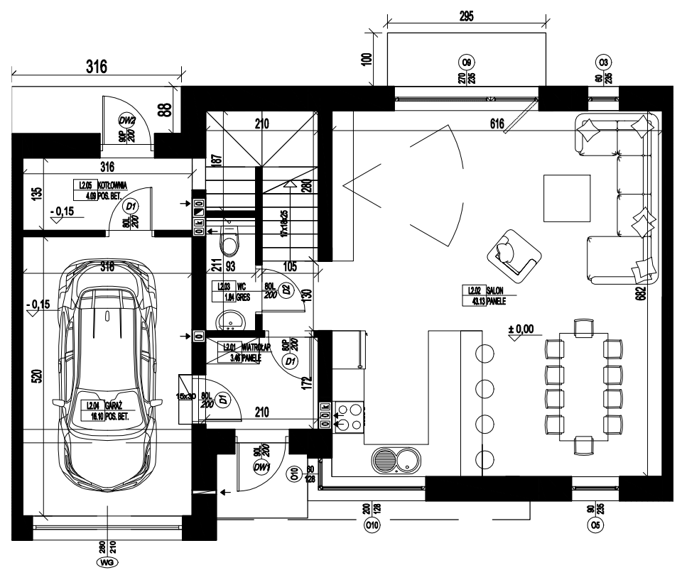
RZUT PARTERU
